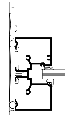
4 ALT. JAMB
