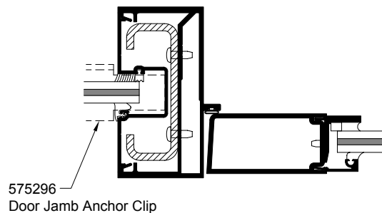
3 DOOR AT JAMB
